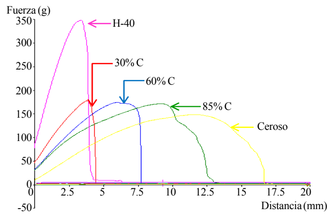
Figura 4. Efecto del incremento de la fracción amilopectina sobre la fuerza de tensión y extensibilidad de la tortilla a 2 h de haber sido elaboradas.
