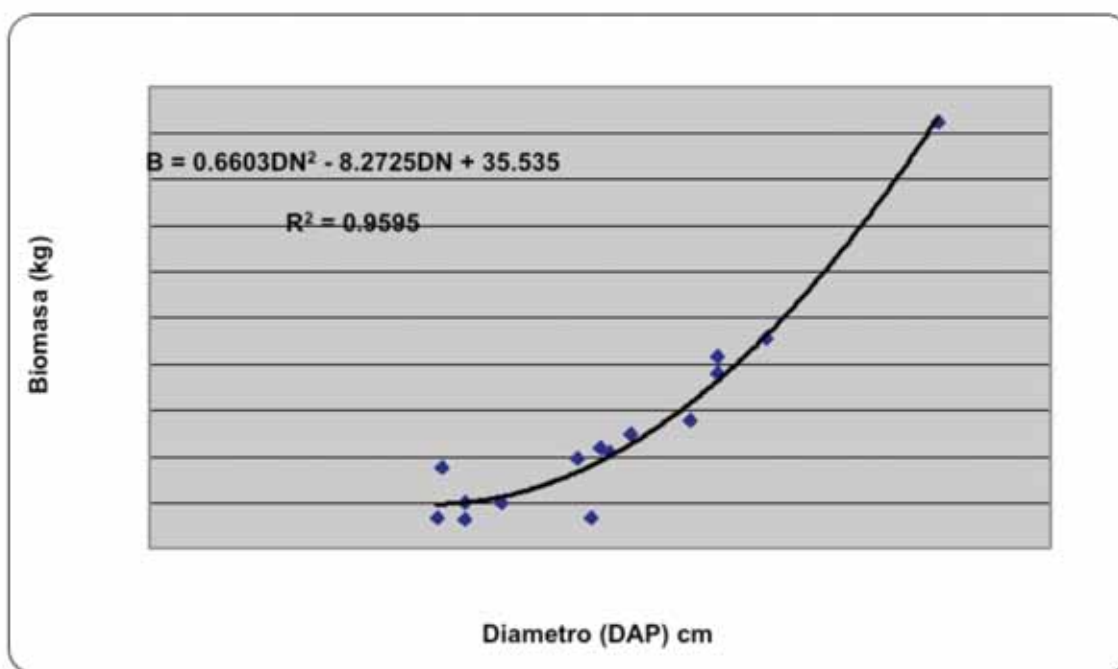
Figura 2. Relación entre el diámetro a la altura del pecho y la biomasa por clase diamétrica en Swietenia macrophylla King. Figure 2. Relation between DBH and biomass by diametric class in Swietenia macrophylla King.
