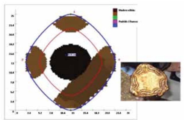
Figura 15. Tomograma ultrasónico de Dicksonia squarrosa (G. Forst.) Sw. para la determinación morfométrica, tamaño del diámetro de los tallos y estado general de sanidad forestal de un espécimen juvenil a la altura del pecho.
