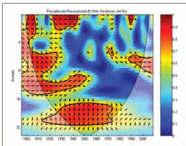
Figura 12. Dominio de coherencia de ondeleta entre la precipitación reconstruida y los índices de ENSO 3.4. Figure 12. Wavelet coherence domain relative to reconstructed precipitation series, and ENSO 3.4 index.
