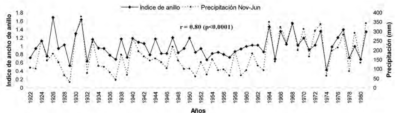
Figura 5. Asociación entre el índice de ancho de anillo y la precipitación regional estacional noviembre-junio para el período común 1922 - 1981.
