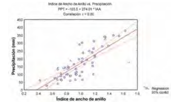
Figura 6. Dispersión del modelo de regresión lineal. Figure 6. Scatter plot and linear regression model.
