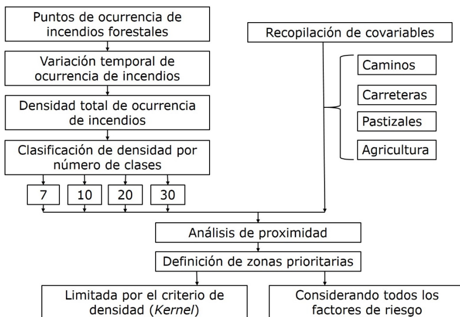
Figura 2. Diagrama de flujo general del proceso metodológico para la clasificación de áreas prioritarias contra incendios forestales.
