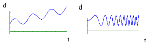
Figura 1. Gráficas senoidales.
