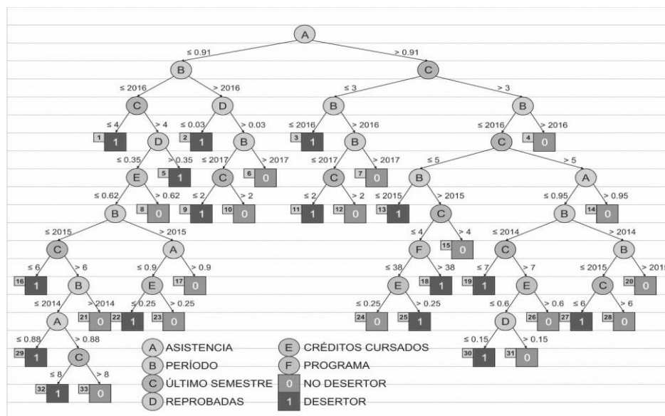
Figura 3. Árbol de decisión C4.5 generado a partir del conjunto de datos de entrenamiento usando las variables obtenidas por el método de selección Relief
