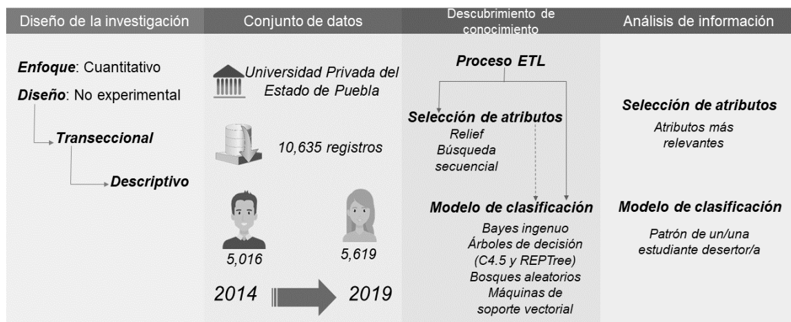
Figura 1. Metodología para determinar los atributos más relevantes en la deserción universitaria
