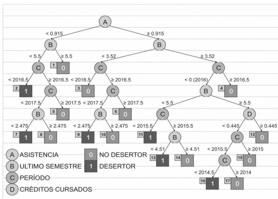
Figura 2. Árbol de decisión REPTree generado a partir del conjunto de datos de entrenamiento usando la totalidad de atributos
