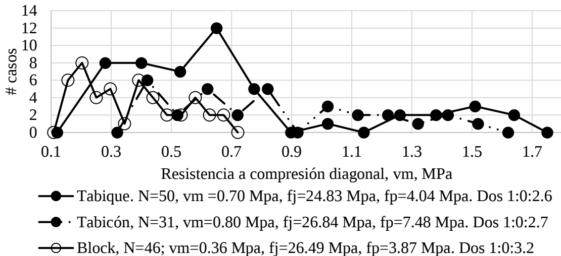
Figura 9. Polígonos de frequência de resistência à compressão diagonal com argamassa de tipo I
