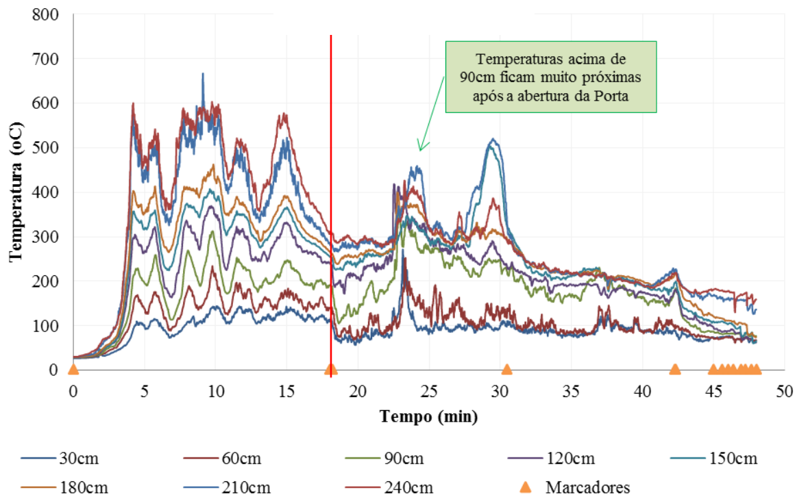
Figura 6. Temperatura aferidas na haste de termopares colocada no centro do compartimento
