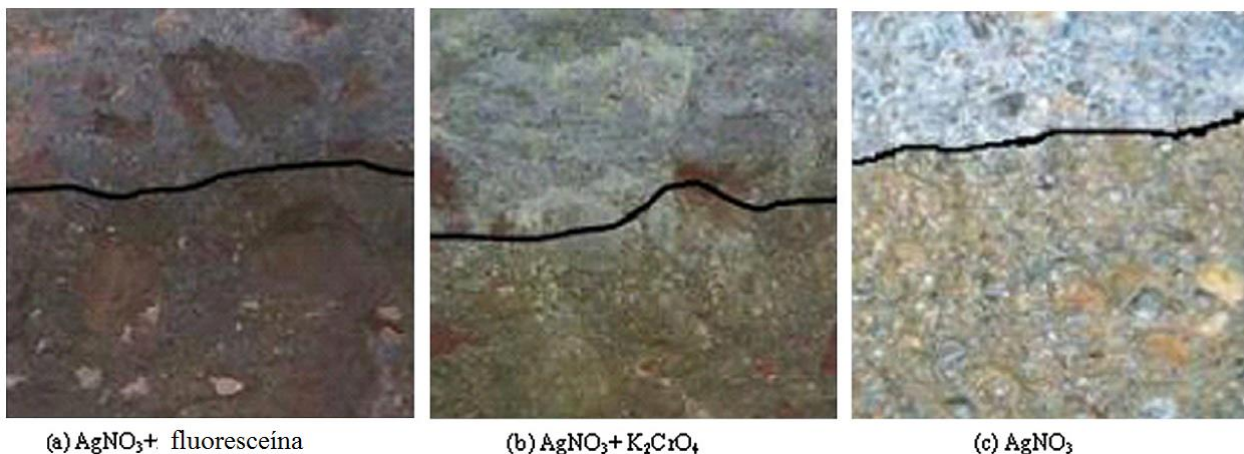
Figura 9. a) \text{AgNO}_3 + \text{fluoresceína} b) \text{AgNO}_3 + \text{K}_2\text{CrO}_4 c) \text{AgNO}_3 (Adaptado de He et al. , 2011).
