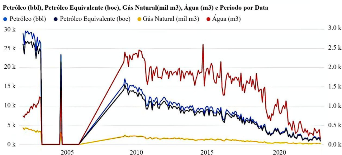
Figura 1. Descenso de la producción en las plataformas petrolíferas de la cuenca de Campos con desmantelamiento aprobado.
