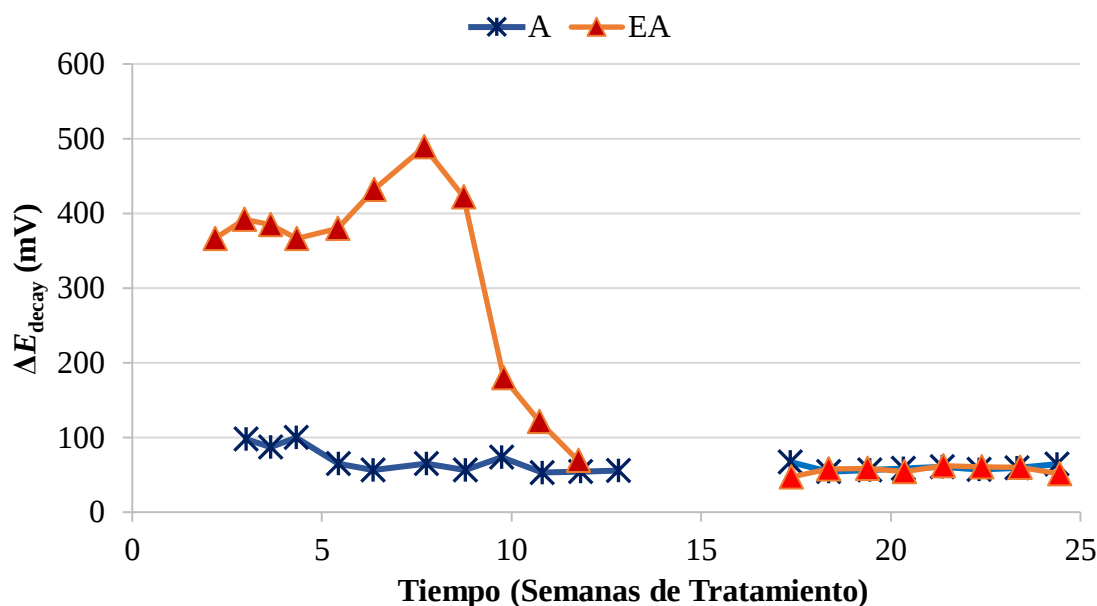
Figura 3. Evolución del \Delta E_{\text{decay}} durante el tratamiento de PC. A: PC; EA: EEC + PC. Todos ellos sometidos a un proceso de contaminación de \text{Cl}^- durante 24 semanas. Los tratamientos electroquímicos fueron interrumpidos desde la semana 13 a la 17. Adaptada de (Carmona, et al., 2015a).
