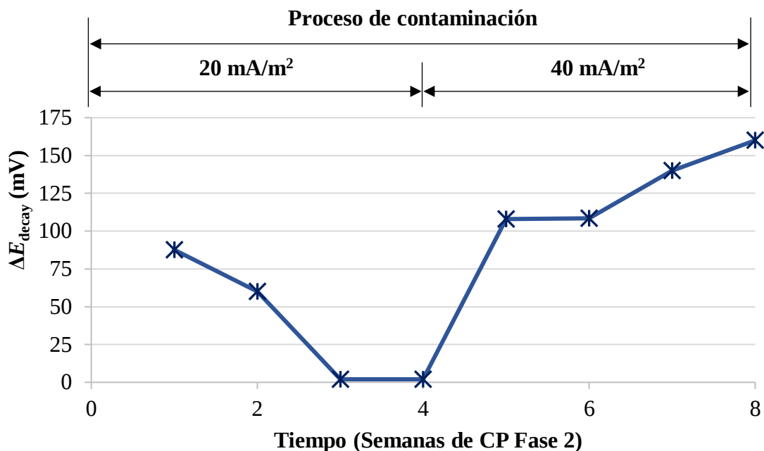
Figura 4. Evolución del \Delta E_{\text{decay}} para la probeta EA (EEC+PC) durante la fase 2. Primera etapa de 4 semanas donde se aplicaron 20 mA/cm 2 , y segunda etapa donde se aplicaron 40 mA/cm 2 .
