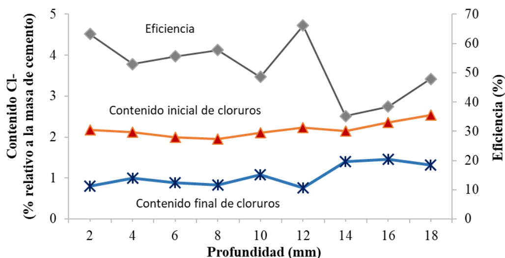
Figura 2. Perfiles de contenido de \text{Cl}^- (eje Y1), correspondientes a los estados antes y después del tratamiento de EEC. En el Y2 se representan las eficiencias locales. Adaptada de (Carmona, et al., 2015a).
