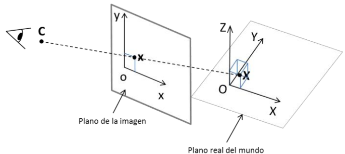
Fig. 3. Modelo “ pinhole ” (o cámara oscura) que representa el plano 2D de la imagen en la cámara con respecto al espacio real 3D del mundo. Un punto X en el espacio real es generado como x en el plano de la cámara. El punto C representa el centro de la cámara [15].
