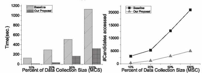
(b) MSC dataset
