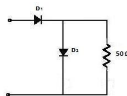
Fig. 12. Conmutador serie-paralelo [6].
