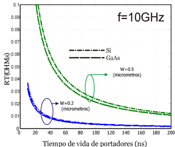
Fig. 7. Respuesta de R_s vs. \tau en diodos p-i-n de Si y GaAs en altas frecuencias.
