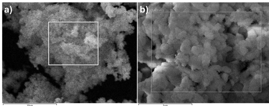
FIGURA 5. Micro áreas de SEM con escala de 5 y 10 \mu\text{m} de: a) CaO, y, b) Sr9/CaO calcinado a 80. 0 ° C.
