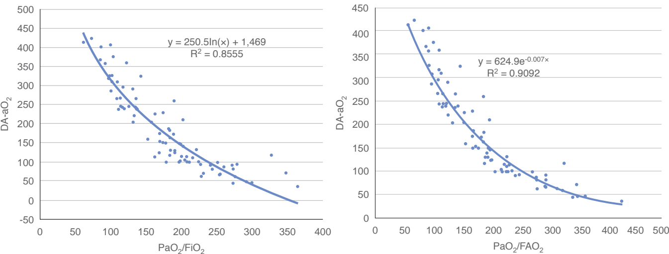
Figura 2: Correlación de la DA-aO 2 con los índices PaO 2 /FAO 2 y PaO 2 /FiO 2 . R 2 = coeficiente de determinación.
