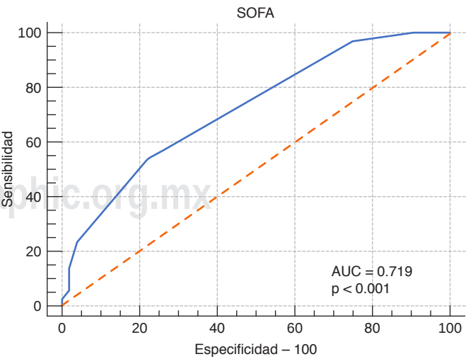
Figura 1: Curva ROC (Receiver Operating Characteristic) de la escala SOFA para predecir el uso de ventilación mecánica invasiva. SOFA = Sequential Organ Failure Assessment, AUC = Área bajo la curva.
