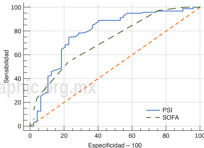
Figura 3: Comparación de curvas ROC de PSI/PORT con SOFA para predecir uso de ventilación mecánica. ROC = Receiver Operating Characteristic, SOFA = Sequential Organ Failure Assessment.
