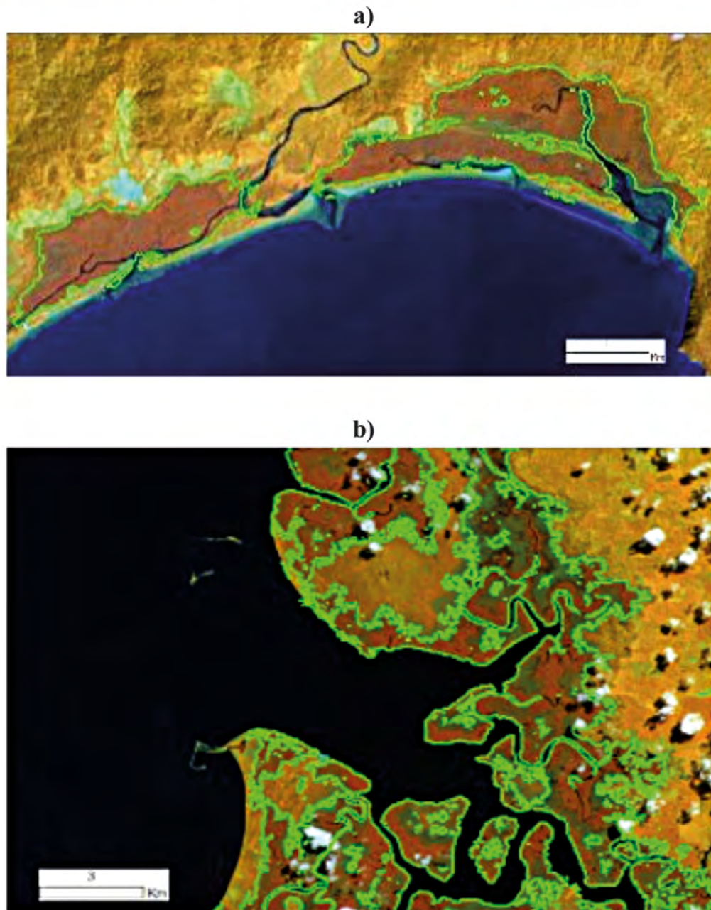
FIGURA 3. Ejemplo de combinaciones espectrales para la identificación de mangle en imágenes Sentinel-2.
