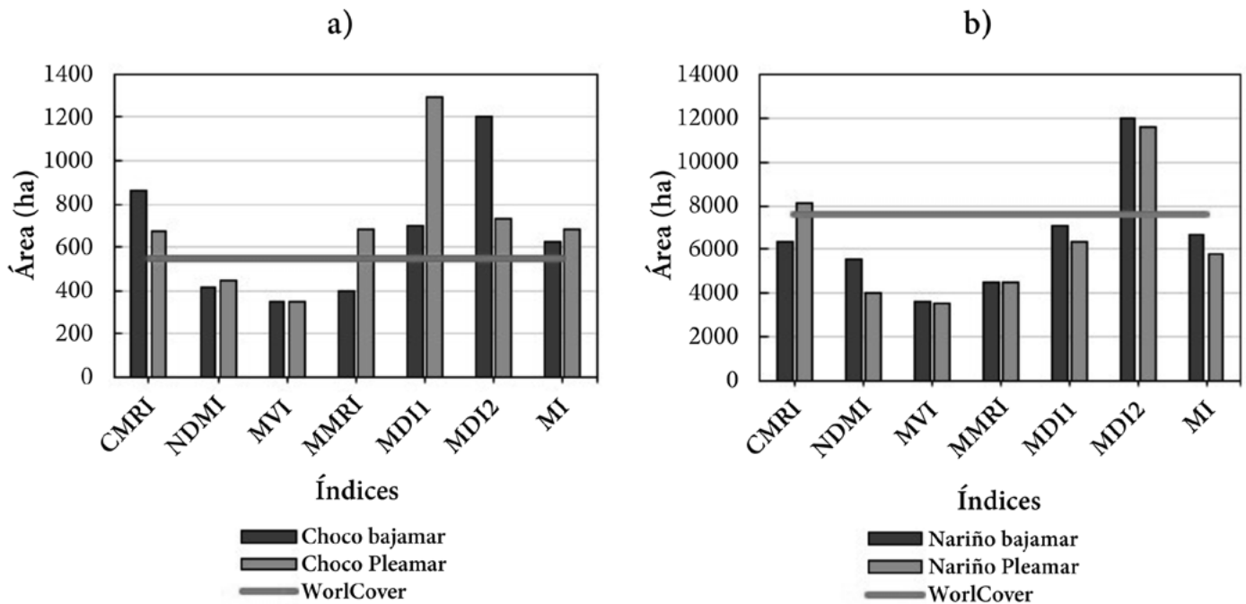
FIGURA 5. Comparación de las áreas de manglares derivadas de los índices de vegetación en a) Chocó y b) Nariño.
