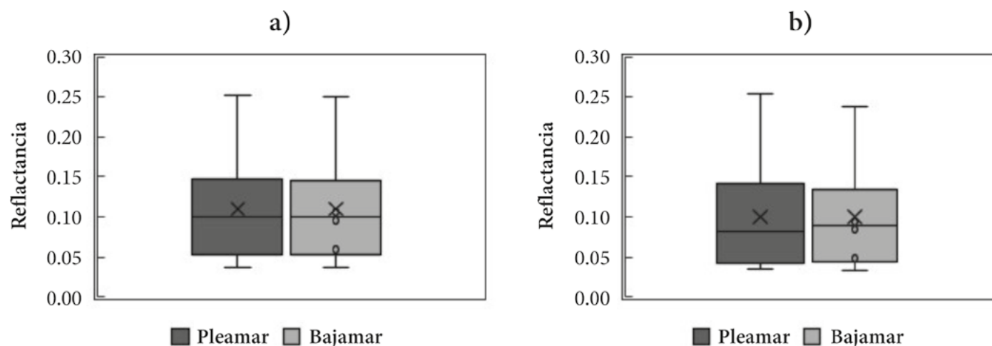
FIGURA 4. Firma espectral promedio de los manglares de Nariño y del Chocó en los diferentes estados mareales, a) Chocó y b) Nariño.
