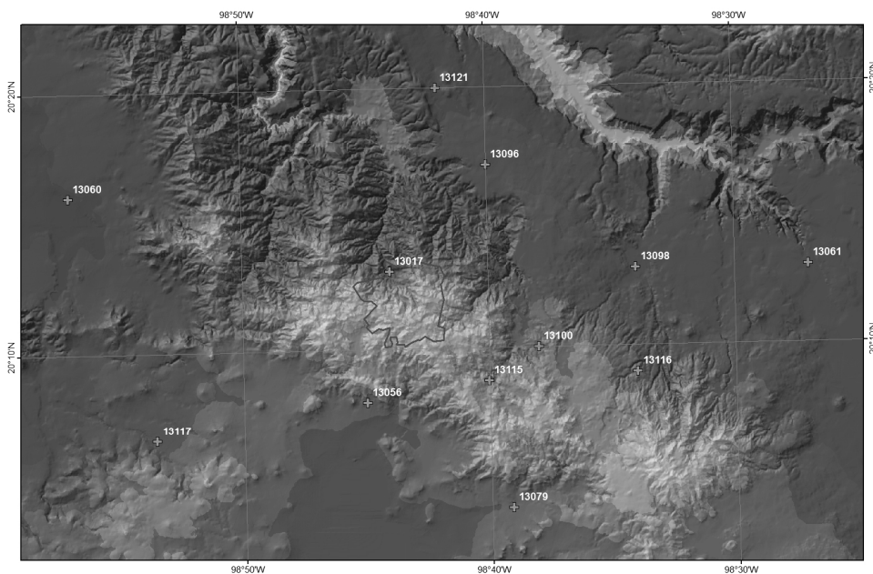
Figura 2. Localización de las estaciones meteorológicas utilizadas.
