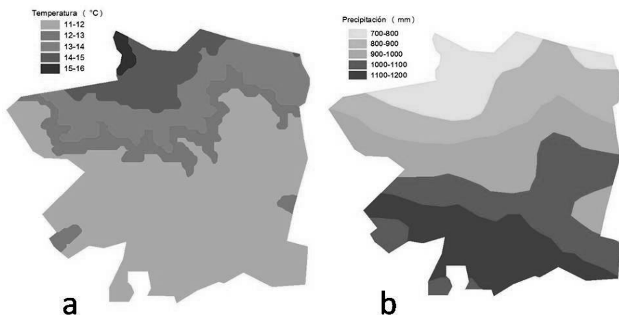
Figura 3. Se muestra en a) la temperatura media anual (°C) y en b) la precipitación promedio anual (mm) obtenida para el parque.
