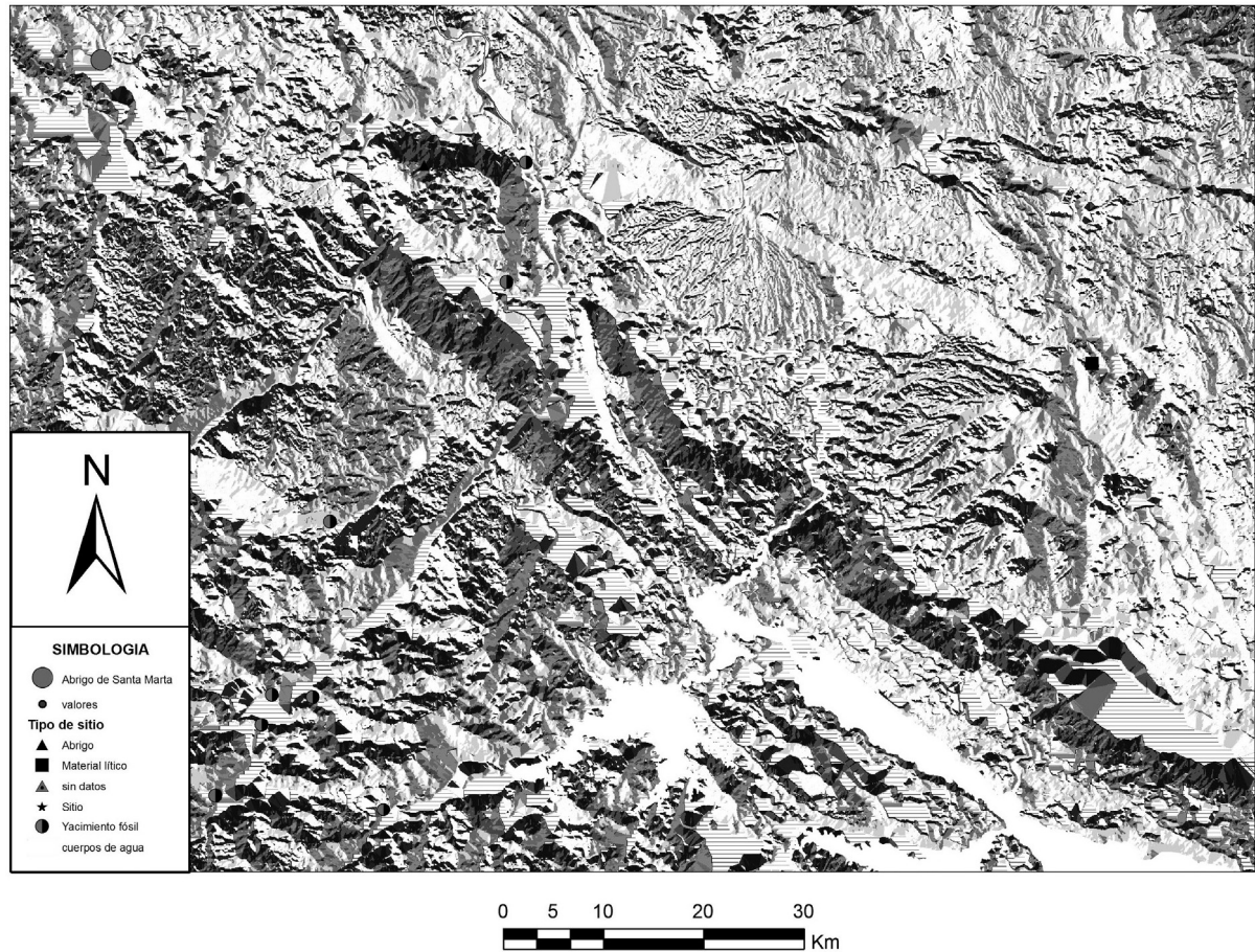
Mapa 5. Proceso de caracterización del DEM y los sitios analizados. DEM que muestra la dirección de las pendientes
