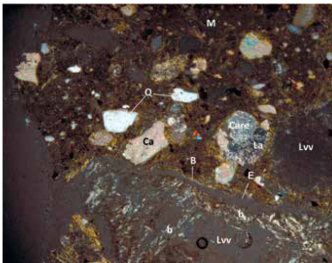
FIGURAS 7 y 8. Microfotografías en luz natural (arriba) y luz polarizada (abajo) de un fragmento de la muestra TG254 en la cual es perceptible un fragmento de roca volcánica vítrea (Lvv) con borde de alteración (B); internamente exhibe huellas de alteración (b), espacio vacío relleno de medio de montaje (E); al exterior de él, formando parte de los desgrasantes, calcita espática (Ca) y cuarzo (Q). En ocasiones fue posible documentar (misma figura al centro) vidrio alterado (La) reemplazado parcialmente por calcita (Care). Ambas microfotografías, tomadas con objetivo 4x (Microfotografías: Víctor M. Dávila, 2014; cortesía: Instituto de Geología [IG-UNAM], México).
