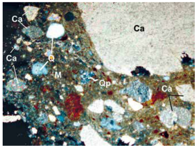
FIGURAS 9 y 10. Microfotografías en luz natural (arriba) y luz polarizada (abajo) de la muestra TG255 que exhiben la relación desgrasantes/matriz. Ca = calcita espática, Q = cuarzo monocristalino, Qp = cuarzo policristalino, Lv = lítico volcánico (?), M = matriz arcillosa. Objetivo 10x (Microfotografías: Víctor M. Dávila, 2014; cortesía: Instituto de Geología [IG-UNAM], México).
