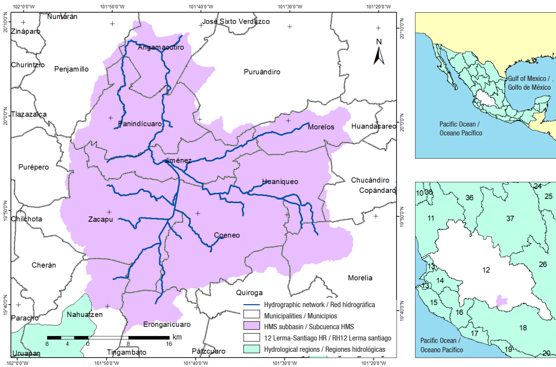
Figure 3. Location of the basin (HEC-GeoHMS). Figura 3. Localización de la cuenca (HEC-GeoHMS).
