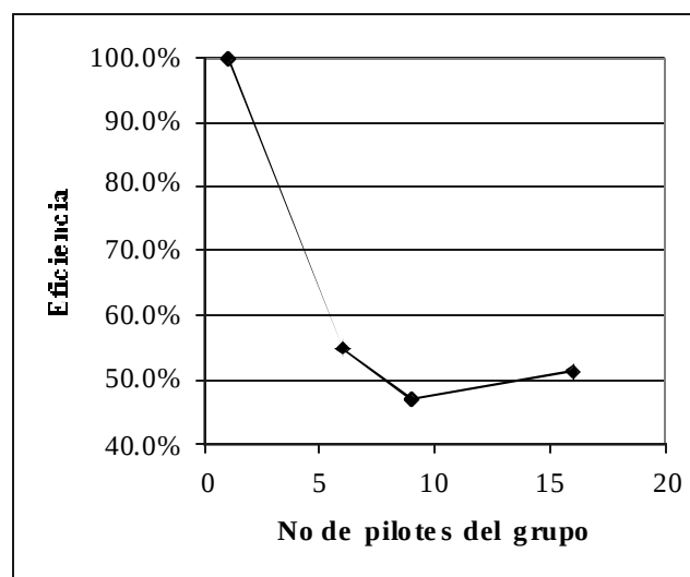
Figura 13. Eficiencia de grupos de pilotes
