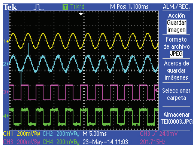
Figura 10. Se muestran en orden descendente las señales del mensaje enviado V_{sb} , del recuperado V'_{sb} , del mensaje enviado V_{sa} y del recuperado V'_{sa} ; todo en funcionamiento bidireccional y en tiempo real F_s = 200\text{Hz}
