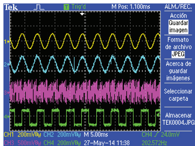
Figura 11. Se muestran en orden descendente las señales del mensaje enviado V_{sb} , del mensaje recuperado V'_{sb} , la señal caótica encriptadora del mensaje V_{sa} y el mensaje recuperado V'_{sa} , en forma bidireccional y en tiempo real F_s = 200\text{Hz}
