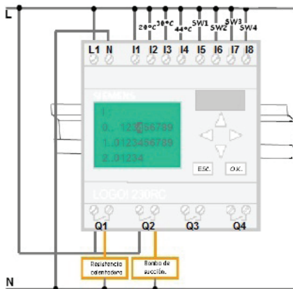
Figura 6. Conexiones externas al PLC, donde I_{2,3,4} entradas de temperatura; I_{5,6,7,8} interruptores de inicio de operación y Q_{1,2}
