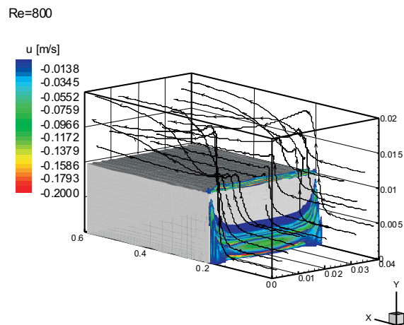
Figura 5. Líneas de corriente y zonas de recirculación para Re=800
