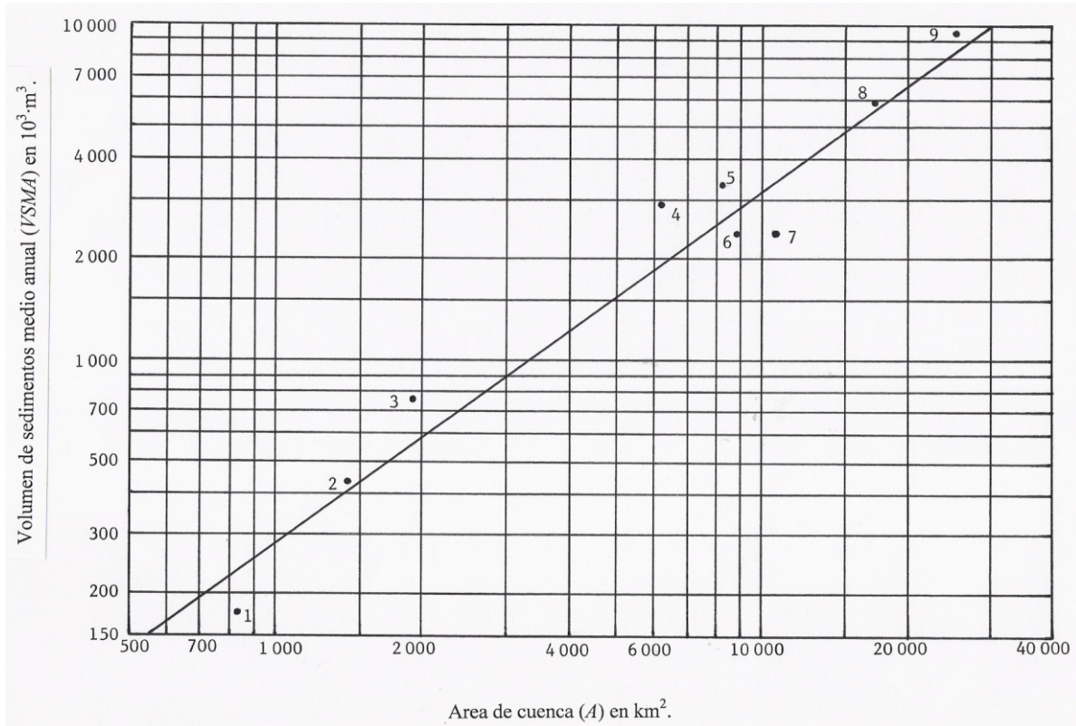
Figura 1. Relación entre el volumen de sedimentos medio anual (VSMA) en miles de m³ y el área de cuenca (A) en km² en la Región Hidrológica Num. 10 (Sinaloa)
