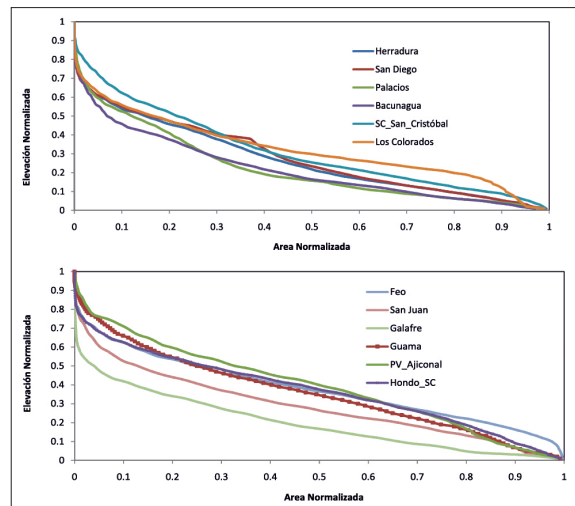
Figura 11. Curvas hipsométricas de los ríos que drenan la llanura sur de Pinar del Río.
