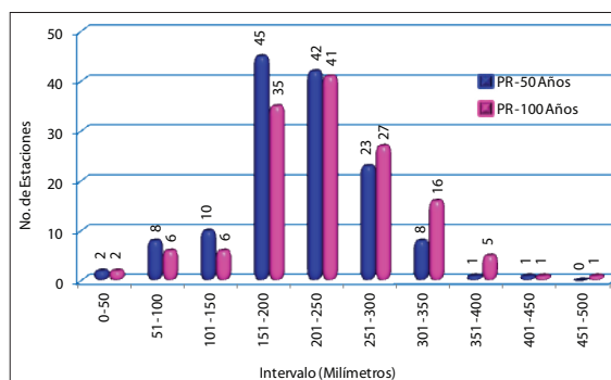
Figura 5. Lluvias torrenciales a nivel anual, a 100 y 50 años de periodo de retorno.
