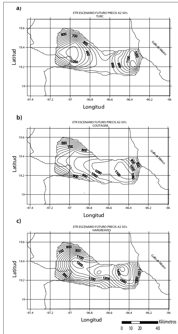
Figura 13. Escenario futuro A2 del comportamiento de la evapotranspiración real (mm/año) para la década de los cincuenta con el modelo PRECIS; a) Fórmula de Turc, b) Fórmula de Coutagne y c) Fórmula de Hargreaves.
