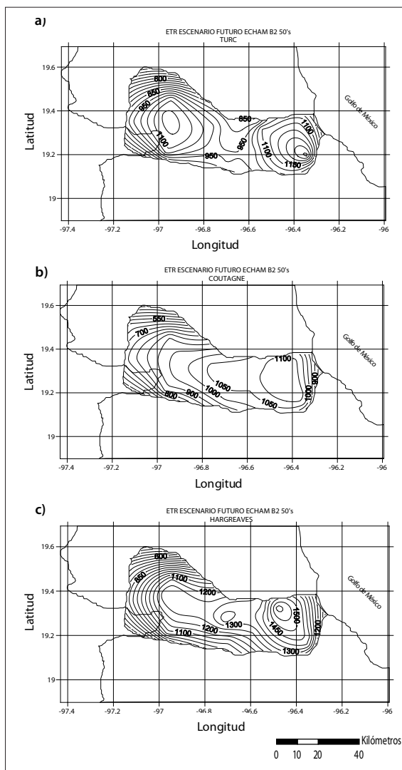
Figura 7. Escenario futuro B2 del comportamiento de la evapotranspiración real (mm/año) para la década de los cincuenta con el modelo ECHAM; a) Fórmula de Turc, b) Fórmula de Coutagne y c) Fórmula de Hargreaves.
