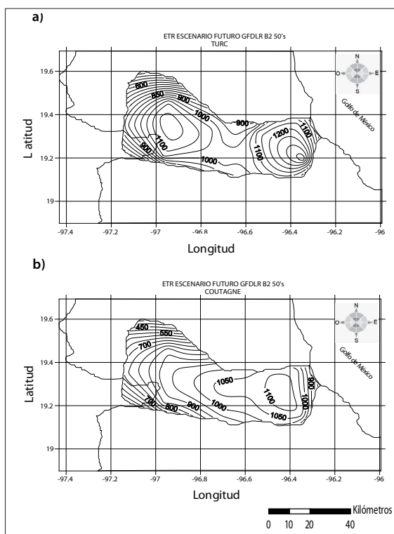
Figura 11. Escenario futuro B2 del comportamiento de la evapotranspiración real (mm/año) para la década de los cincuenta con el modelo GFDLR; a) Fórmula de Turc, b) Fórmula de Coutagne.
