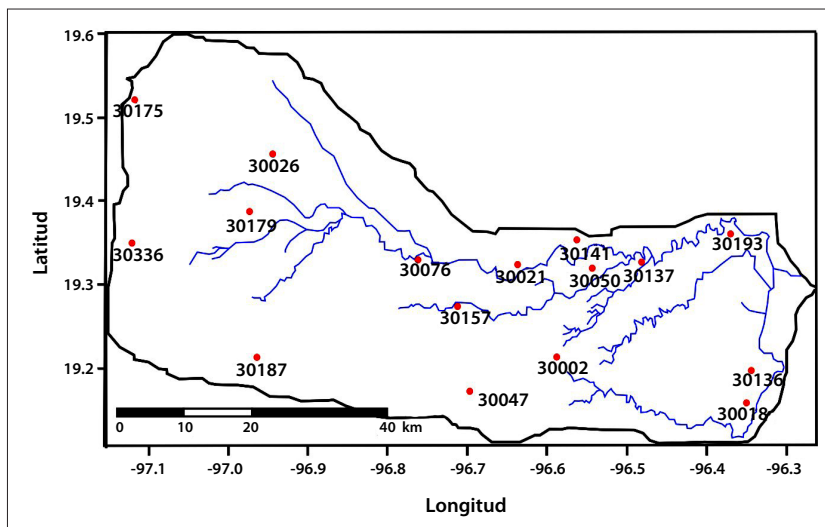
Figura 2. Estaciones climatológicas ubicadas en la cuenca del río La Antigua (tomada de CONAGUA, 2001 y modificada por Pereyra et al. , 2008).
