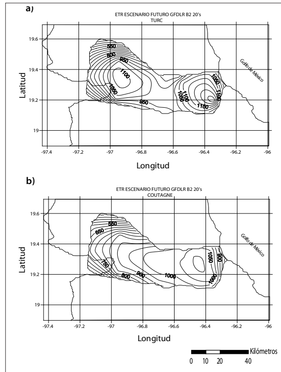
Figura 9. Escenario futuro B2 del comportamiento de la evapotranspiración real (mm/año) para la década de los veinte con el modelo GFDLR; Fórmula de Turc, Fórmula de Coutagne.
