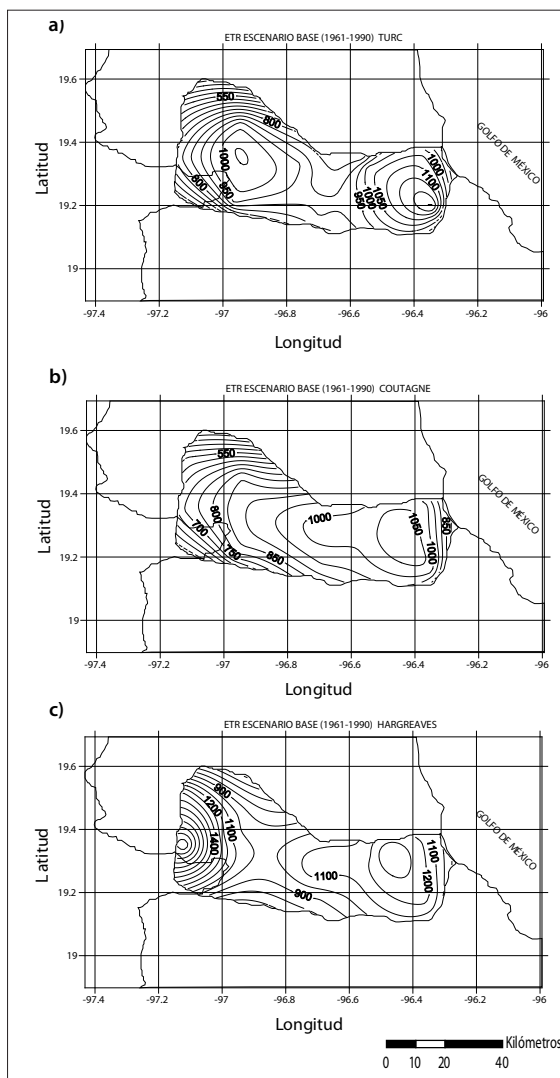
Figura 3. Escenario base del comportamiento de la evapotranspiración real (mm/año) utilizando: a) Turc, b) Coutagne y c) Hargreaves, a partir de la Normales Climatológicas 1961-1990.
