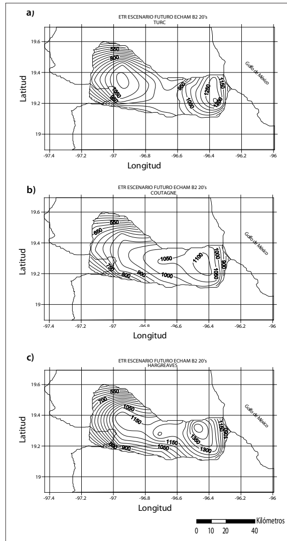
Figura 5. Escenario futuro B2 del comportamiento de la evapotranspiración real (mm/año) para la década de los veinte con el modelo ECHAM; a) Fórmula de Turc, b) Fórmula de Coutagne y c) Fórmula de Hargreaves.
