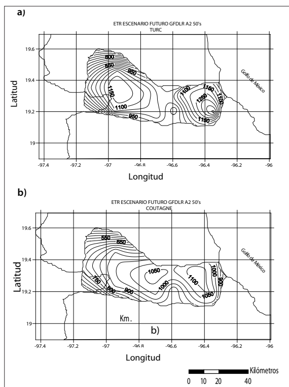
Figura 10. Escenario futuro A2 del comportamiento de la evapotranspiración real (mm/año) para la década de los cincuenta con el modelo GFDLR; a) Fórmula de Turc y b) Fórmula de Coutagne.
