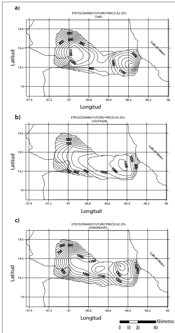
Figura 12. Escenario futuro A2 del comportamiento de la evapotranspiración real (mm/año) para la década de los veinte con el modelo PRECIS; a) Fórmula de Turc, b) Fórmula de Coutagne y c) Fórmula de Hargreaves.
