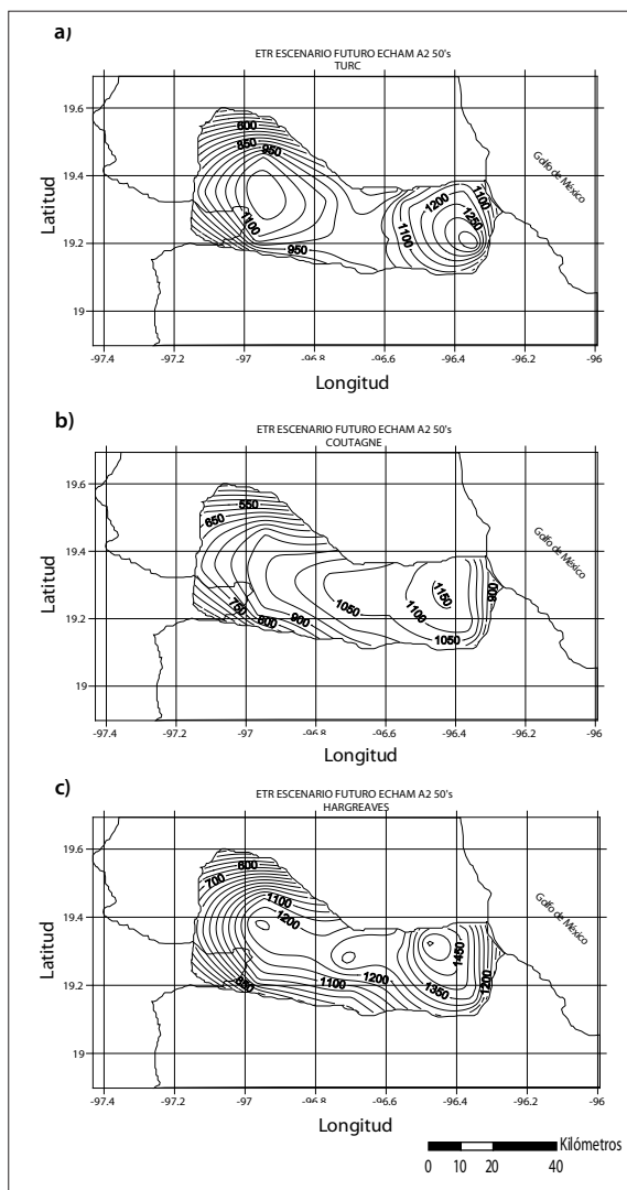
Figura 6. Escenario futuro A2 del comportamiento de la evapotranspiración real (mm/año) para la década de los cincuenta con el modelo ECHAM; a) Fórmula de Turc, b) Fórmula de Coutagne y c) Fórmula de Hargreaves.
