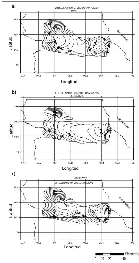
Figura 4. Escenario futuro A2 del comportamiento de la evapotranspiración real (mm/año) para la década de los veinte con el modelo ECHAM.
