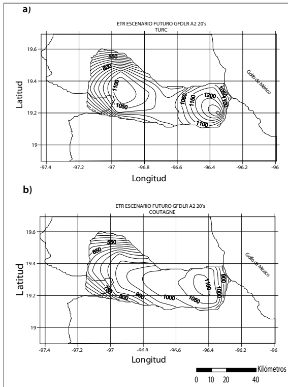
Figura 8. Escenario futuro A2 del comportamiento de la evapotranspiración real (mm/año) para la década de los veinte con el modelo GFDLR; a) Fórmula de Turc y b) Fórmula de Coutagne.
