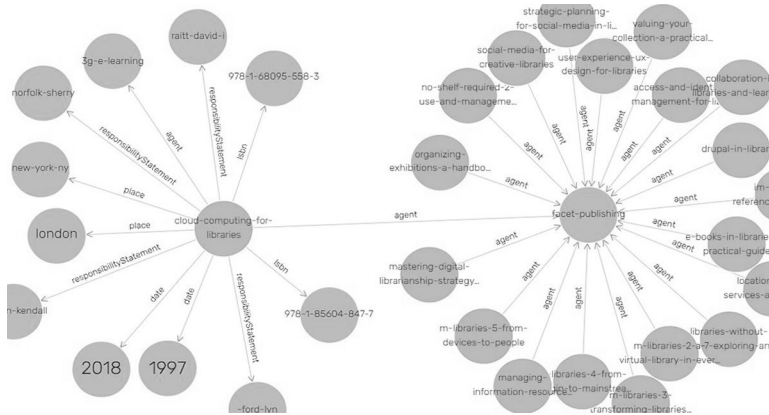
Figura 3. Grafo RDF derivado de la consulta con SPARQL Fuente: elaboración propia, 2020.
