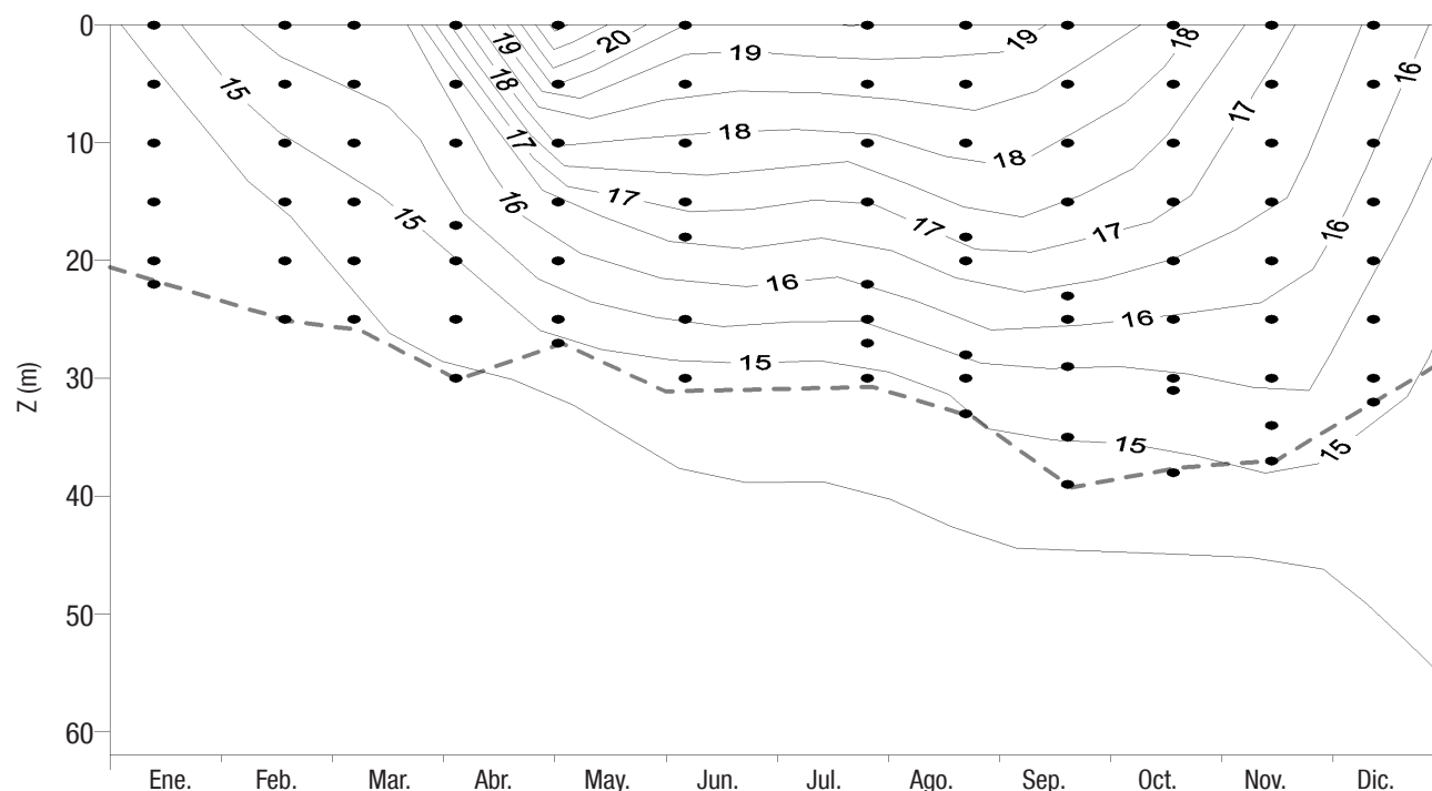
Figura 2. Diagrama pro fundidad-tiempo de isotermas (°C) en el Lago Alchichica, Puebla, México,. El límite de la Zona Eufótica se representa con la línea punteada y las profundidades de incubación con puntos.
