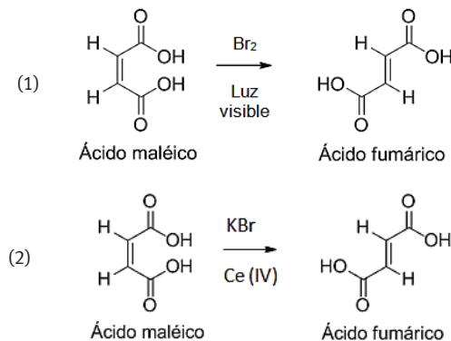
Figura 2. Rutas alternativas (1) y (2) de obtención de ácido fumárico.
