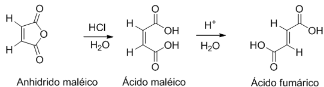
Figura 1. Ruta tradicional de obtención de ácido fumárico.
