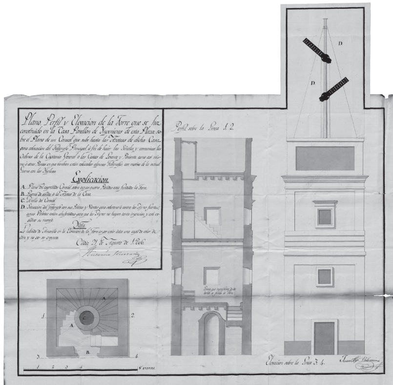
Figura 2. Modelo de las torres y telégrafos ópticos puesto en funcionamiento por el teniente Hurtado en Cádiz. Fuente: Archivo General Militar de Segovia, 50, 535
