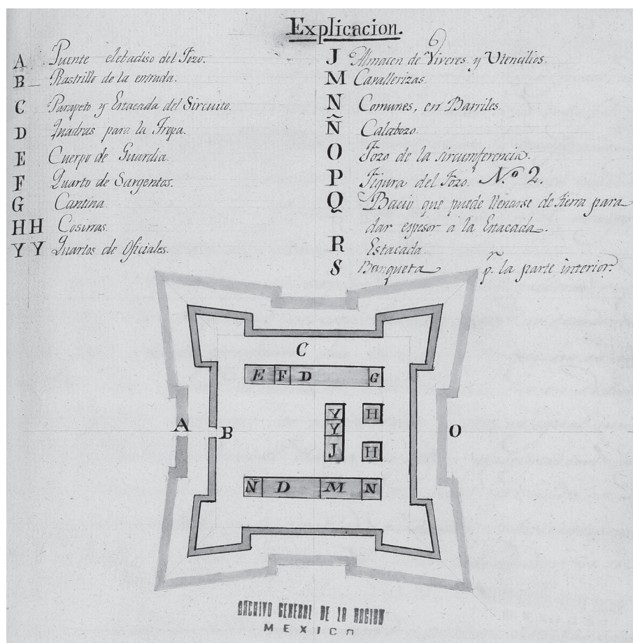
Figura 4. Diseño de la casa fuerte de Santa Fe (fragmento).
