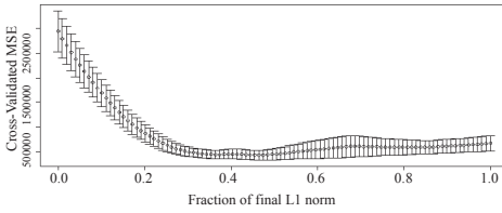
Figura 5 Curva de CV para la variable PMMR1
