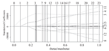
Figura 8 Trayectoria de regularización para la variable PMBCR1
