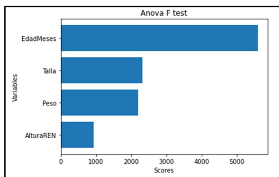
Fig. 2. Comparación de puntuaciones de las características numéricas en el Filtro Anova F-test
