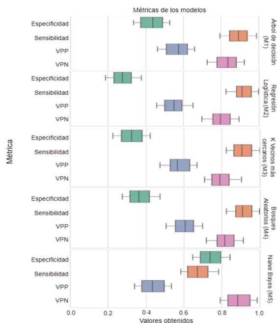
Fig. 4. Diagrama de cajas y bigotes de las métricas
