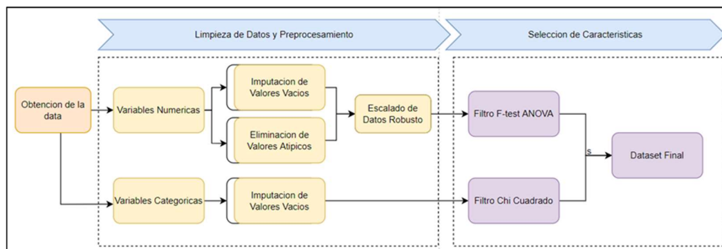
Fig. 1. Metodología propuesta para el modelamiento
