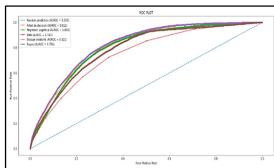
Fig. 6. Gráfica de las curvas ROC de los modelos procesados
