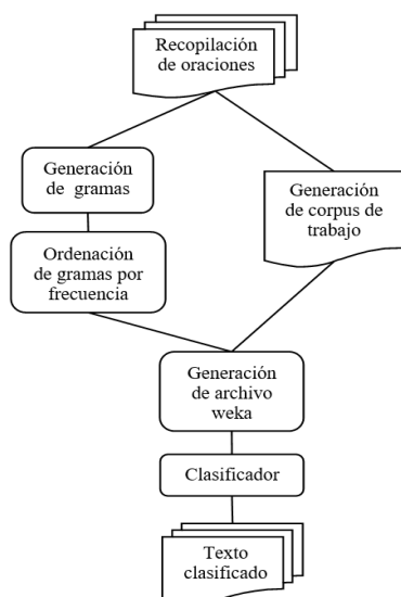
Fig. 1. Modelo propuesto para la identificación de género de textos cortos
