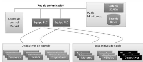
Fig. 1. Representación esquemática del funcionamiento de un Sistema SCADA
