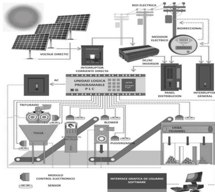
Fig. 3. Infografía de la producción de grava y polvo de vidrio mediante energía solar, controlado por un sistema informático
