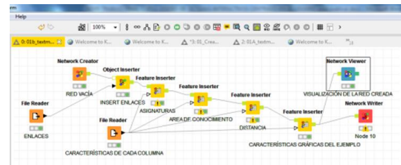
Fig. 16. Secuencia de módulos que permite presentar información en forma de un grafo o red
