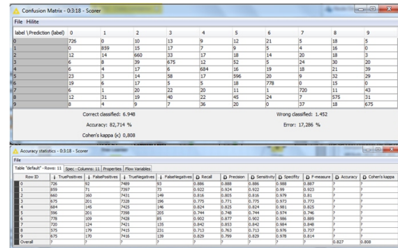
Fig. 9. Matriz de confusión y medidas de exactitud
