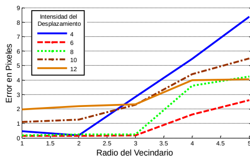
Fig. 4. Gráfica del RMSE de la estimación del desplazamiento en una secuencia corta para validar el algoritmo. El ruido ha sido inducido como un desplazamiento en el plano. Se ha variado la intensidad del desplazamiento y el radio del vecindario de las características candidatas. Los radios y las intensidades están expresados en píxeles
