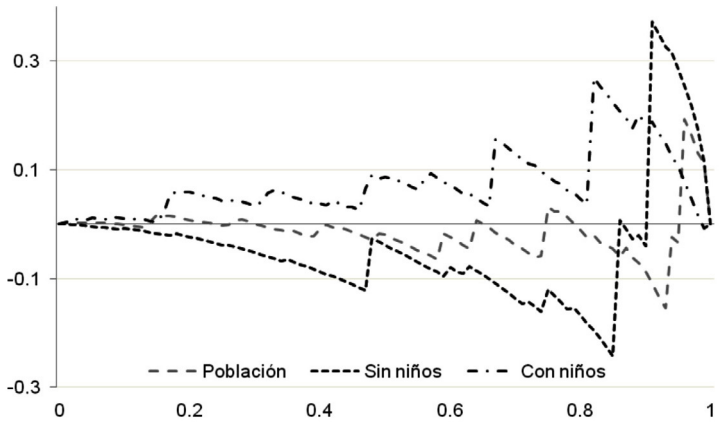
Figura 8. Curvas de progresividad de las Becas en México para hogares con y sin niños, 2010. Fuente: Estimación propia con la base de datos de la ENIGH, 2010.
