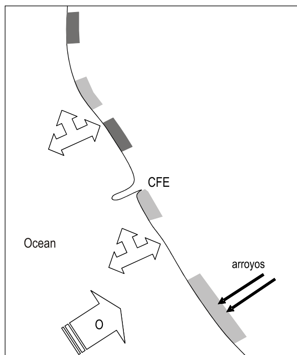
Figura 8. Esquematación fuera de escala de zonas preferenciales de erosión (gris oscuro) y de acreción (gris claro) debidas a la acción del oleaje (flecha O) y el transporte litoral inducido por el mismo (flecha de tres puntas).
