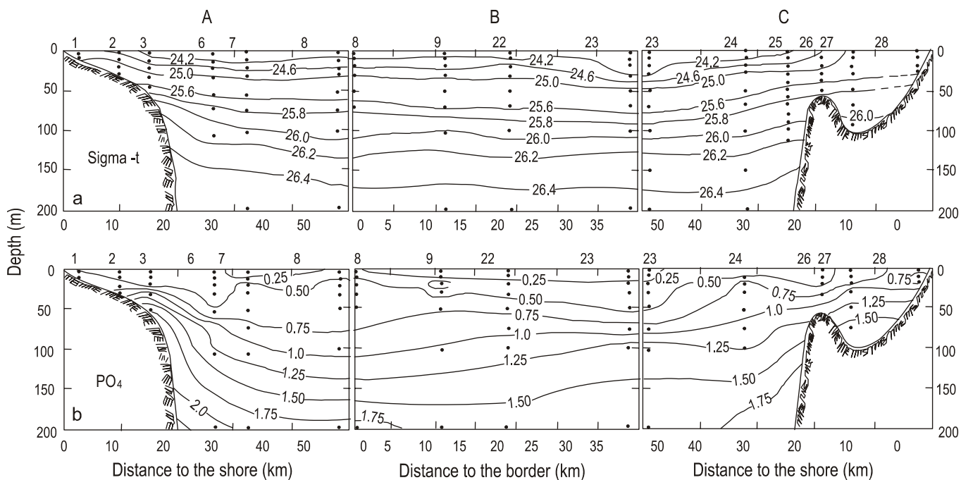
Figura 5. Distribución vertical de (a) densidad y (b) PO 4 3- (μM). El transecto A es el lado norte, el transecto B es el lado paralelo y a 50 km de la costa, y el transecto C es el lado sur (ver fig. 1).
