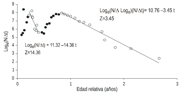
Figura 5. Curva de captura linealizada de Pinctada imbricata del banco ostrícola de Guamachito, Península de Araya, Estado Sucre, Venezuela, para la determinación de la mortalidad natural ( Z ) en dos grupos de datos de longitud: (○) datos incluidos en la regresión; (●) datos excluidos de la regresión.
