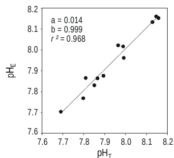
Figura 7. Correlación lineal entre los valores del pH espectrofotométrico ( pH_E ) y pH potenciométrico ( pH_T ) para un conjunto de muestras de aguas estuáricas.
