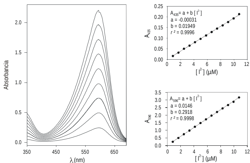
Figura 2. Espectros de absorción de la forma I^{2-} del indicador, obtenidos a pH 11.5 tras adiciones sucesivas de 25 \mu L de azul de timol 2 mM a 60 mL de disolución. Se muestran las regresiones lineales de la concentración del indicador con la absorbancia para la posición de su máximo (596 nm) y a la longitud de onda del máximo de la especie HI^- (435 nm).
