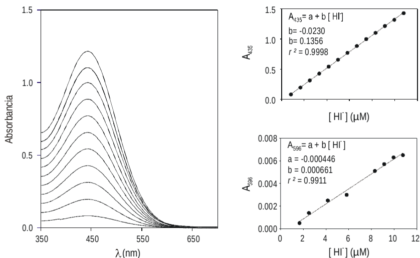
Figura 3. Espectros de absorción de la forma HI^- del indicador obtenidos a pH 5.0 tras adiciones sucesivas de 25 \mu L de azul de timol 2 mM a 60 mL de disolución. Se muestran las regresiones lineales de la concentración del indicador con la absorbancia para la posición de su máximo (435 nm) y a la longitud de onda del máximo de la especie I^{2-} (596 nm).
