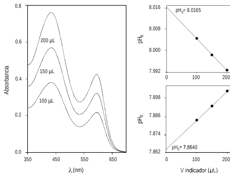
Figura 6. Espectro de absorción de una muestra de 60 mL de agua estuárica ( S = 25.023 , T = 20^\circ C ) tras adiciones de 100, 150 y 200 \mu L de azul de timol 2 mM. A la derecha, se muestran dos ejemplos típicos de cálculo de pH_E inicial de las muestras a partir de las absorbancias a 596 y 435 nm obtenidas después de cada adición de indicador. Figure 6. Absorption spectrum of a 60-mL sample of estuarine water ( S = 25.023 , T = 20^\circ C ) after additions of 100, 150 and 200 \mu L of 2-mM thymol blue. The right-hand plots correspond to two typical examples of the calculation of the initial pH_E of the samples based on absorbances at 596 and 435 nm obtained after each addition of the indicator.
