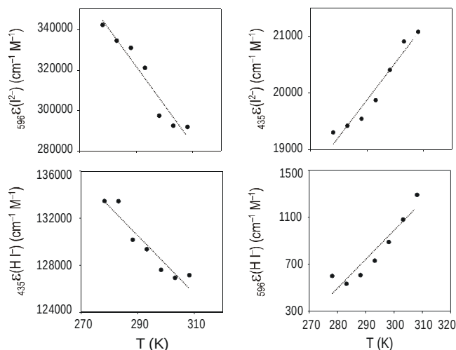
Figura 4. Dependencia de los coeficientes de extinción molar del azul de timol de la temperatura (fuerza iónica 0.5207 M_w ).
