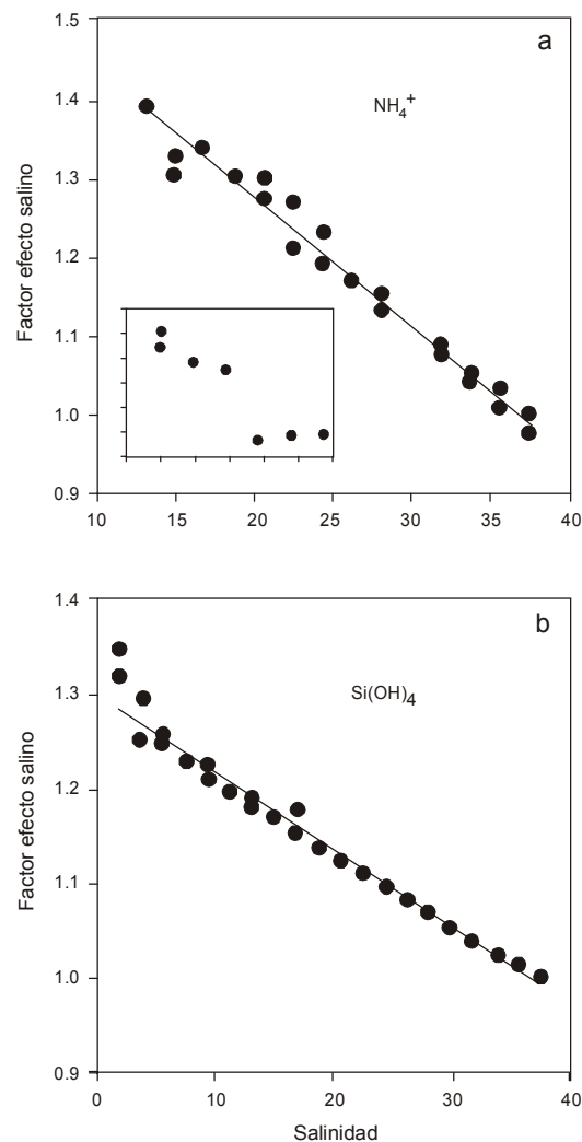
Figura 2. Variación en el "factor efecto salino" con la salinidad para la determinación de amonio (a) y silicatos (b).
