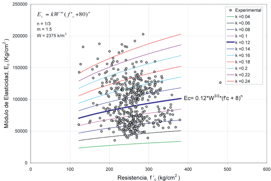
Fig. 10. Análisis de sensibilidad del parámetro k en la ecuación propuesta por la CEC.
