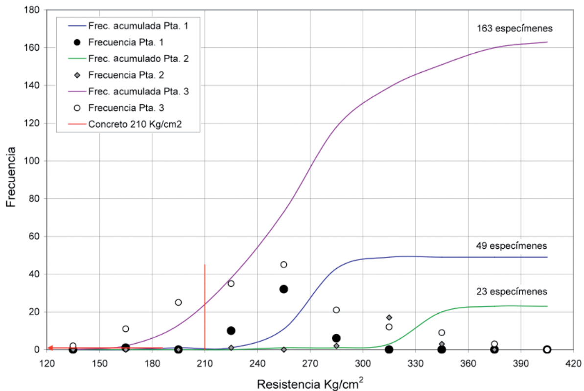
Fig. 3. Resistencia del concreto a los 28 días, muestras con asentamiento de 4 pulgadas.
