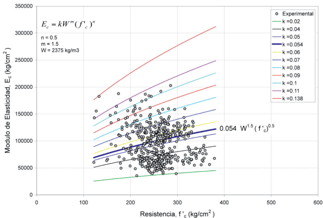
Fig. 9. Análisis de sensibilidad del parámetro k en la ecuación propuesta por el ACI.
