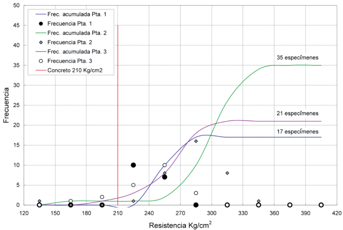
Fig. 5. Resistencia del concreto a los 28 días, muestras con asentamiento de 5 pulgadas.
