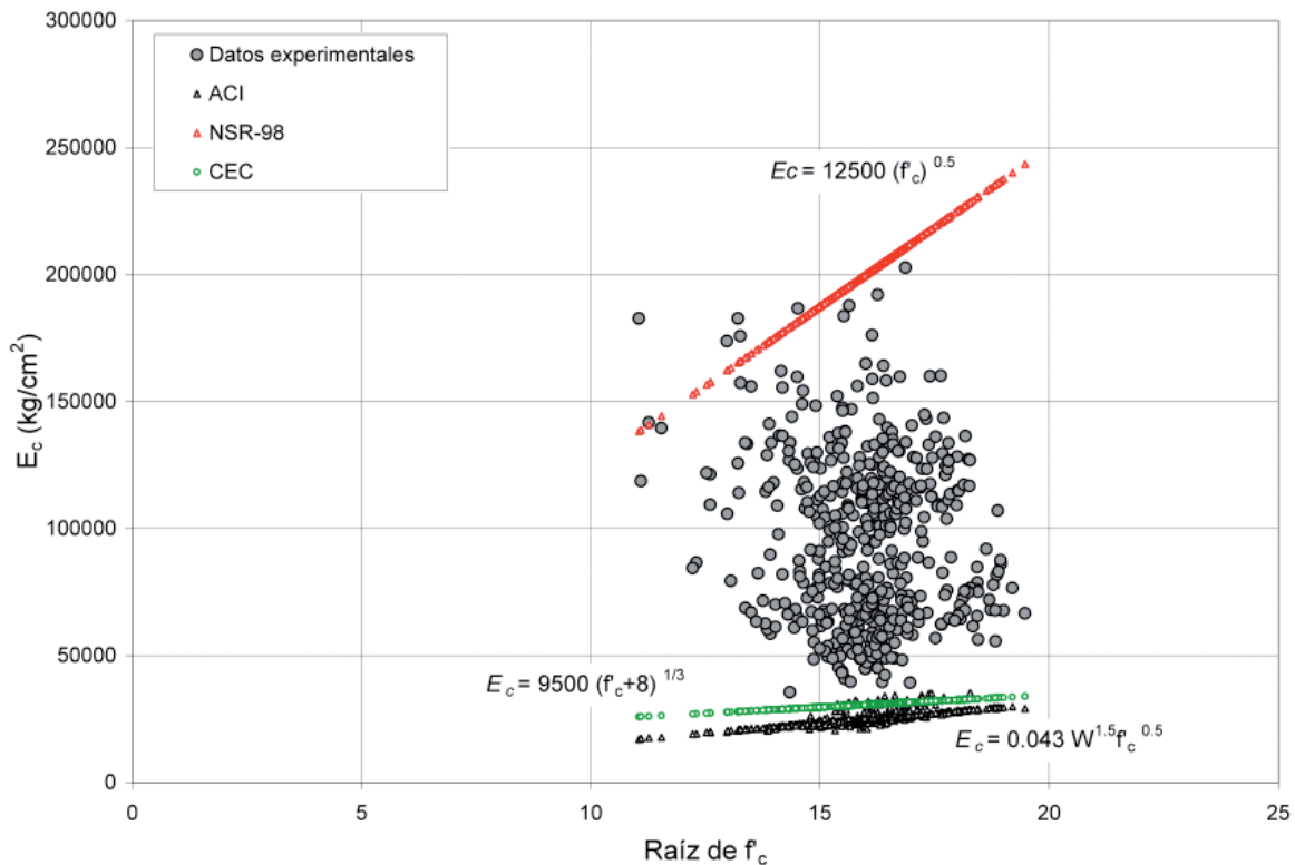
Fig. 6. Comparación del Módulo de Elasticidad Experimental con los valores resultantes al aplicar las ecuaciones propuestas por el ACI, NSR-98 y CEC.
