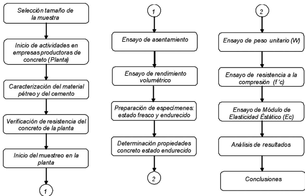
Fig. 2. Metodología seguida para el estudio.
