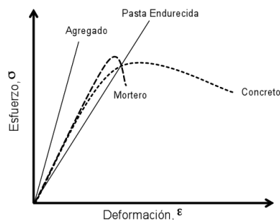
Fig. 1. Relación esfuerzo-elongación en agregado, pasta, mortero y concreto (Adaptada: Topcu y Ugurlo, 2007).
