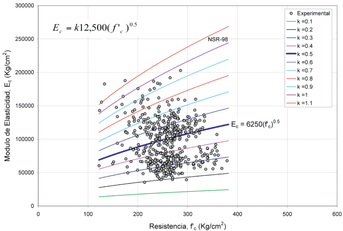
Fig. 7. Análisis de sensibilidad del parámetro k en la ecuación propuesta por el NSR-98.
