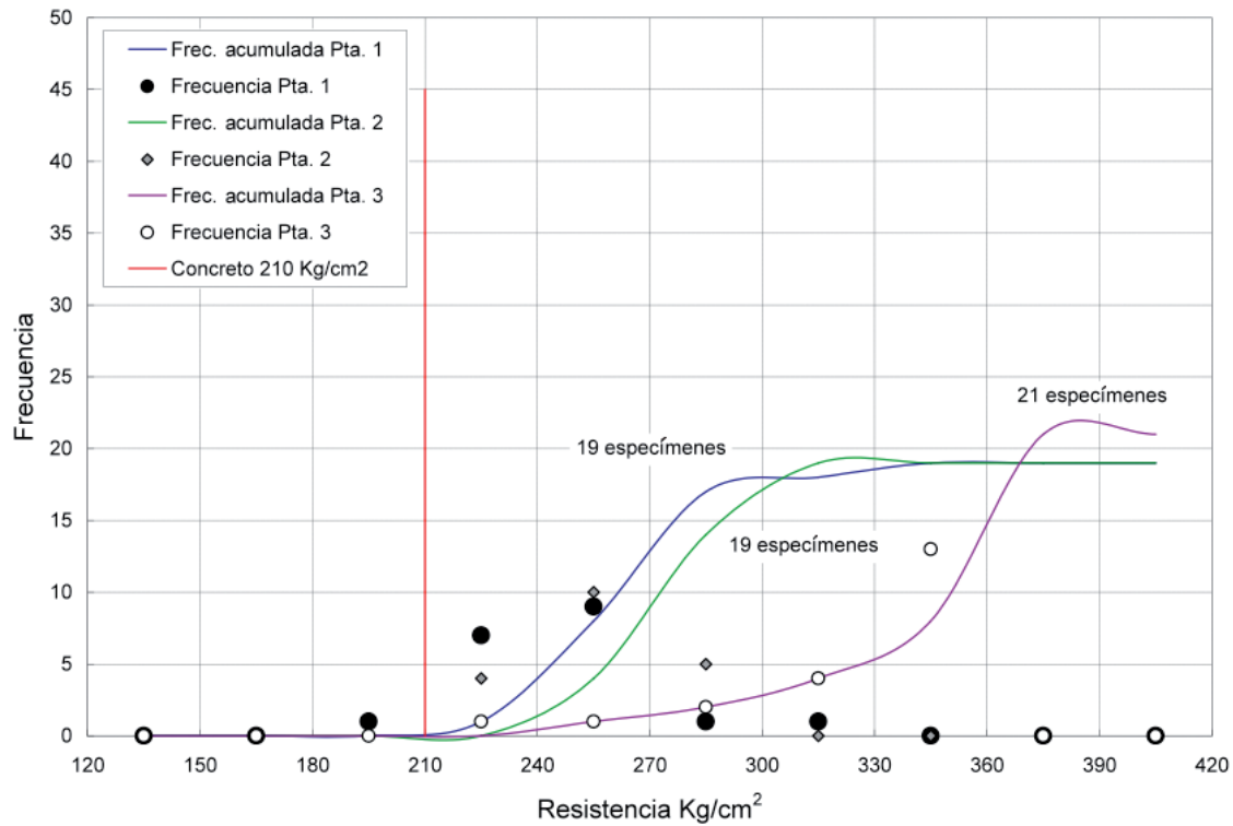
Fig. 4. Resistencia del concreto a los 28 días, muestras con asentamiento de 5 pulgadas.
