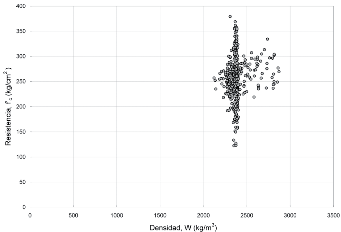
Fig. 8. Variación de la resistencia con la variación del peso unitario del concreto.
