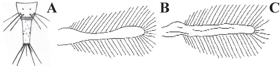
Figura 1. Tubulifera. A Tergo X (tubo) (redibujado de Palmer et al. , 1989). B-C Alas de Phlaeothripidae, B: ala anterior de Karnyothrips . C: ala anterior de Liothrips (Tomadas de Soto-Rodríguez & Retana-Salazar, 2003).
