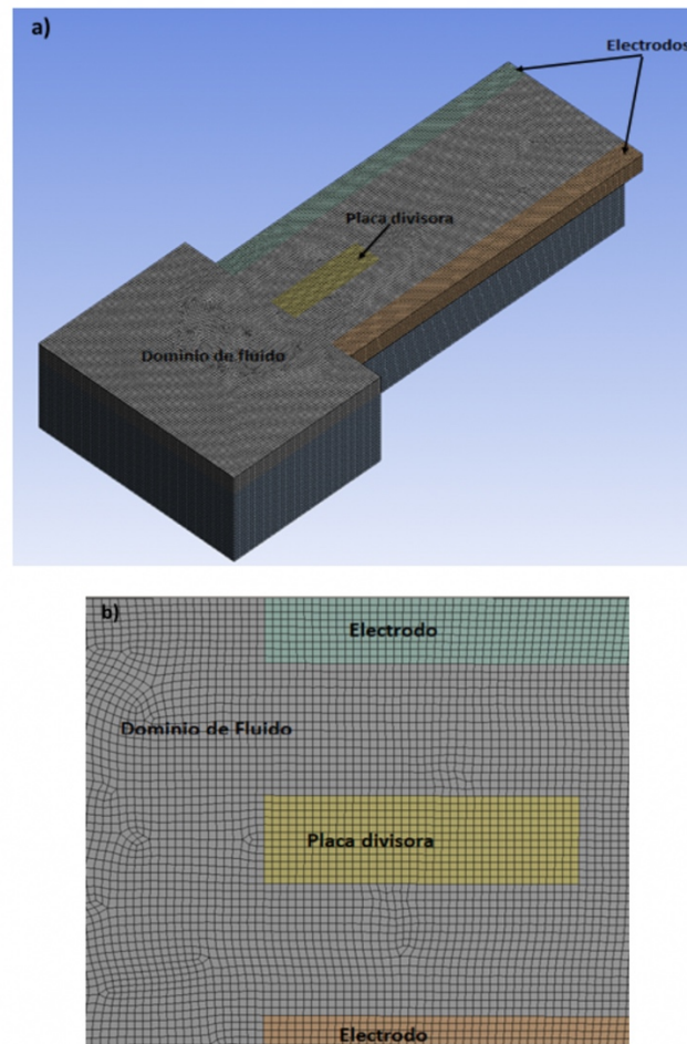
Figura 8. a) Malla generada para el análisis. Sección transversal de corte de la malla realizada en ANSYS Meshing . b) Malla generada para el análisis. Vista a detalle de una sección de la malla generada.
